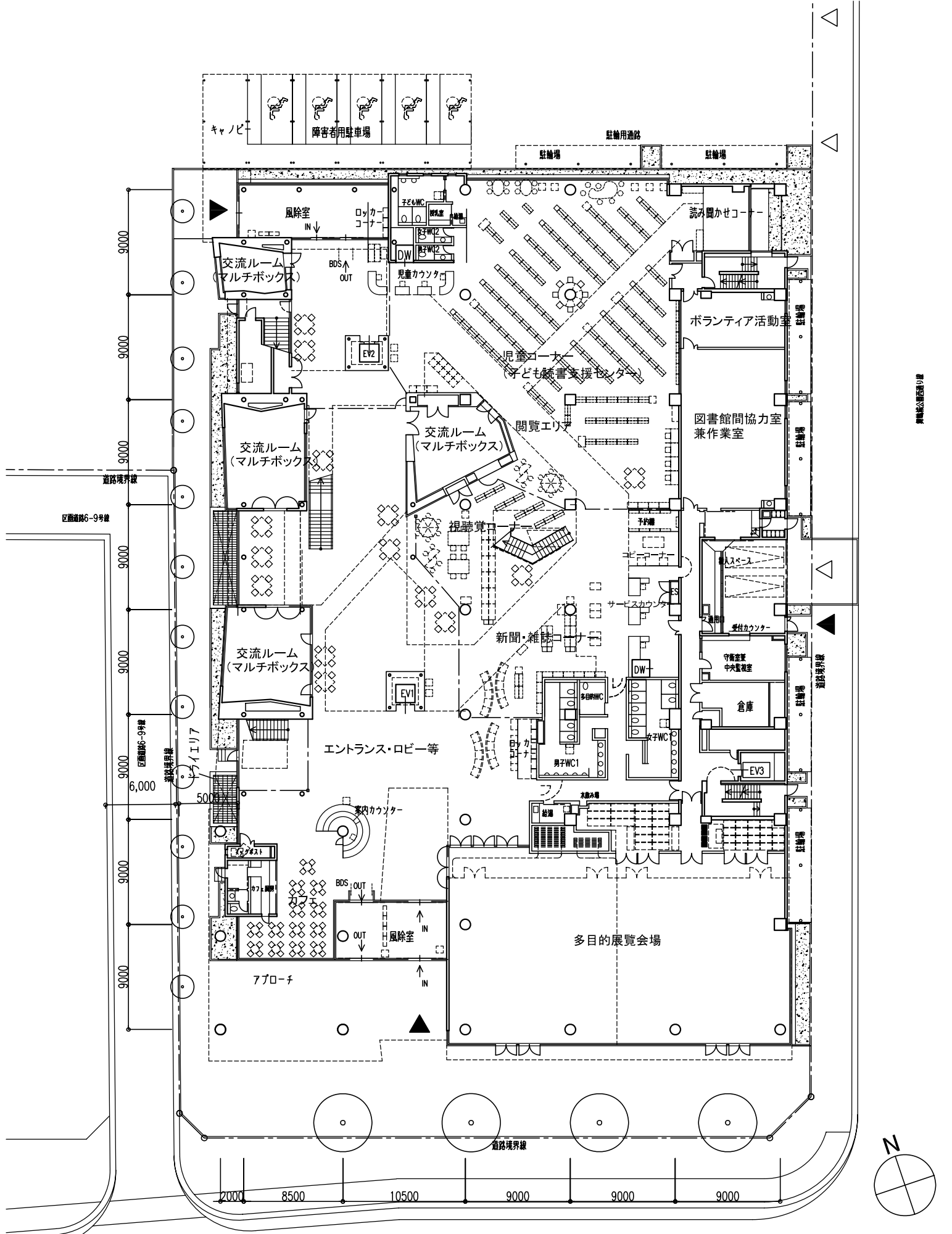
1階平面図
